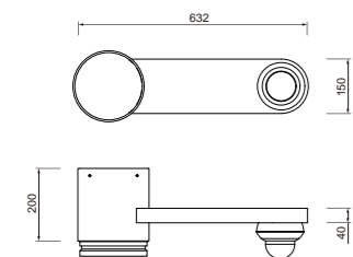
通用摄像头
