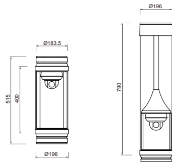
360°摄像头
